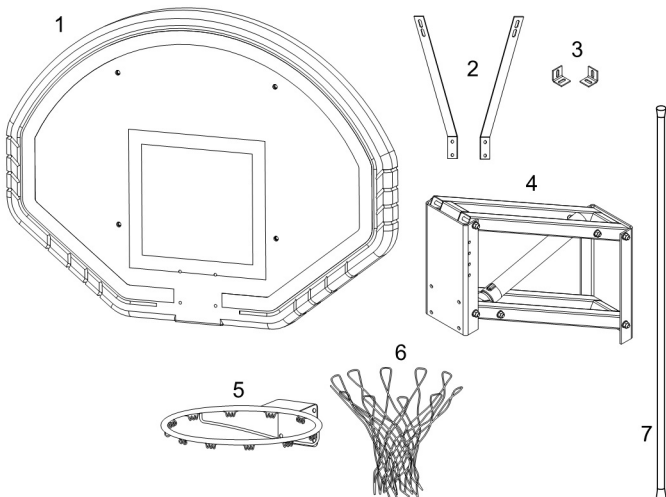
Wykaz części / Parts check list
